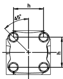
Widok A (DN15-32)
