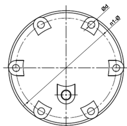
Widok A (DN125-300)
