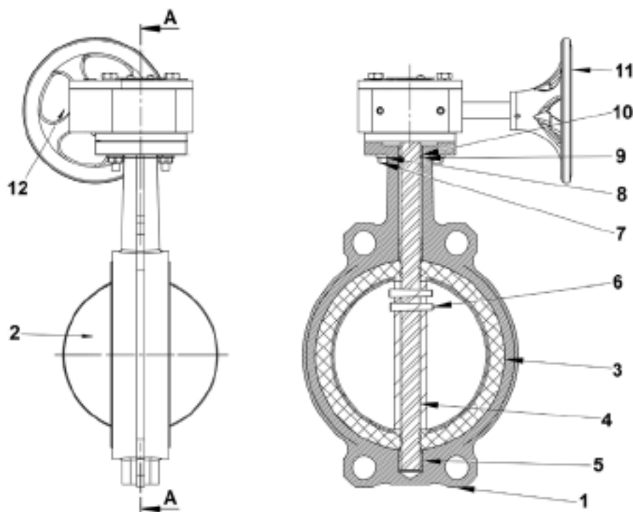
Rzut A-A
